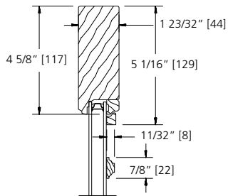
7/8" GRILLE BAR
