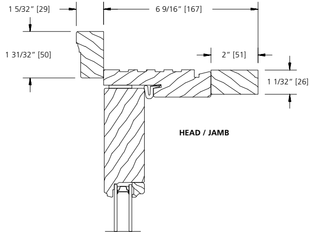
2" OPTIONAL WOOD JAMB EXTENDER (6 9/16" JAMB)
