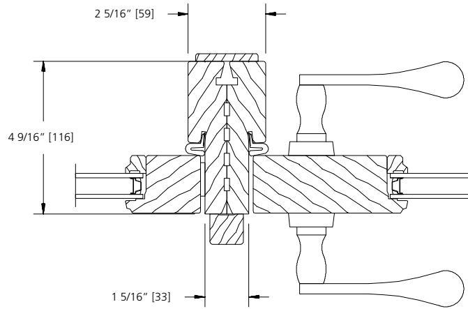
SIDE JAMB
