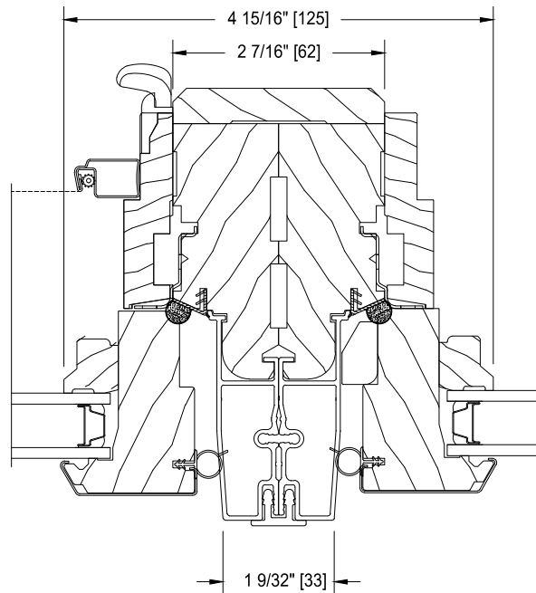
SIDE JAMB
