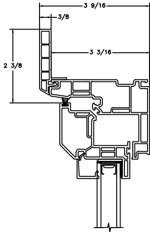
1 5/8" FLUSH FIN
