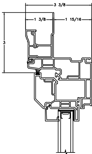
BRICKMOULD
