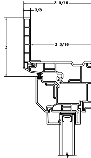
2 1/8" FLUSH FIN
