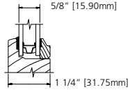
DH INSULATED GLASS
