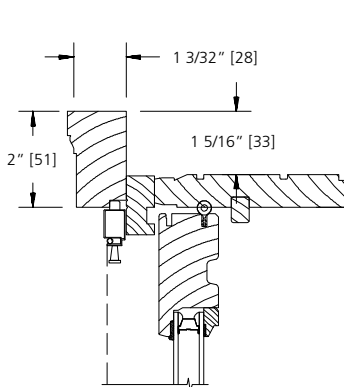
BRICKMOLD
